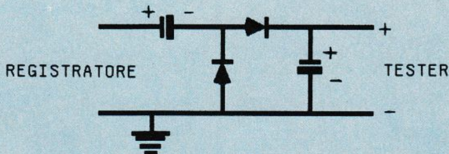
Figura 4. Schema del raddrizzatore-duplicatore.
